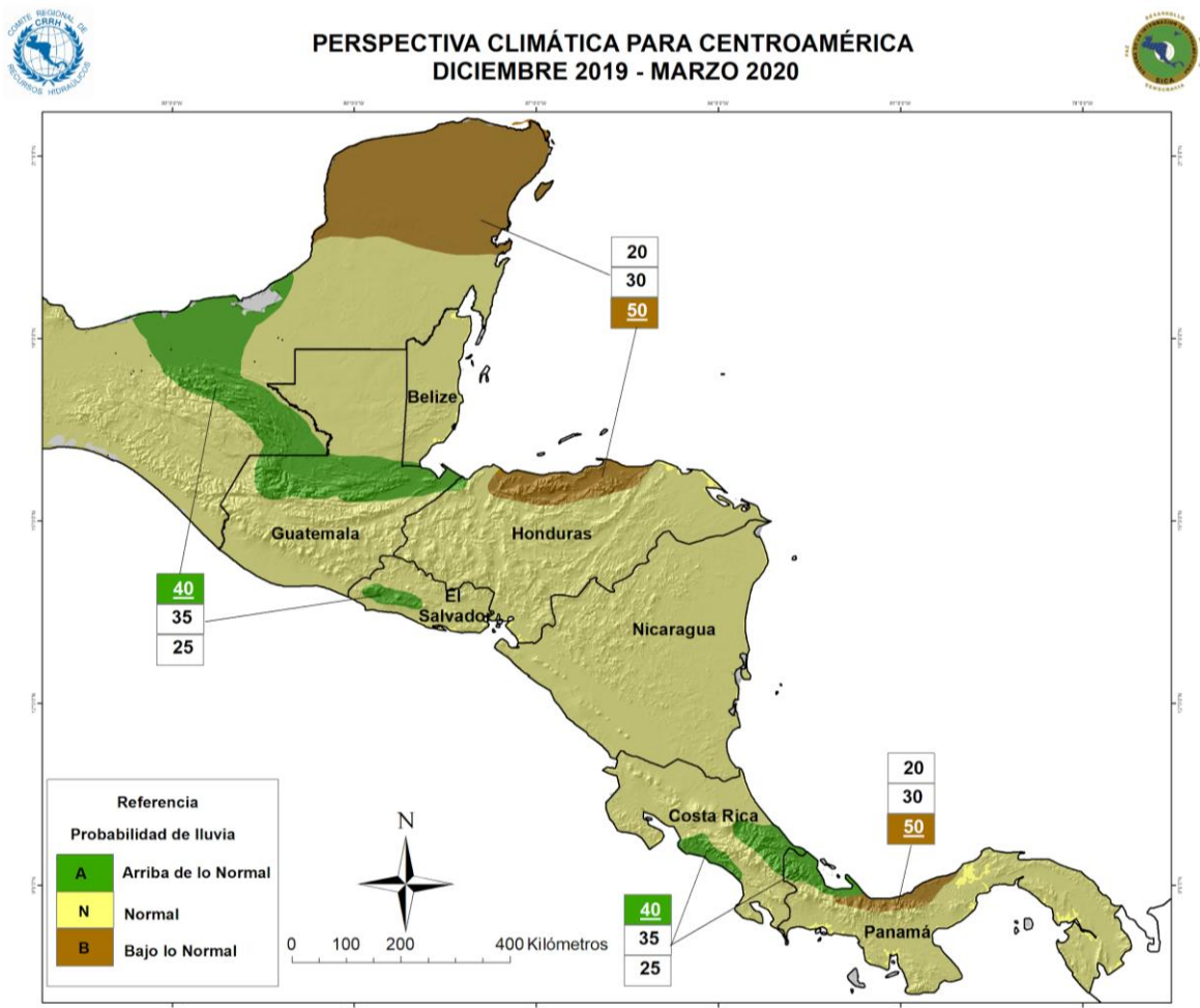
Figura 1. Mapa de la Perspectiva del Clima para Centroamérica y México, diciembre 2019 y marzo 2020
