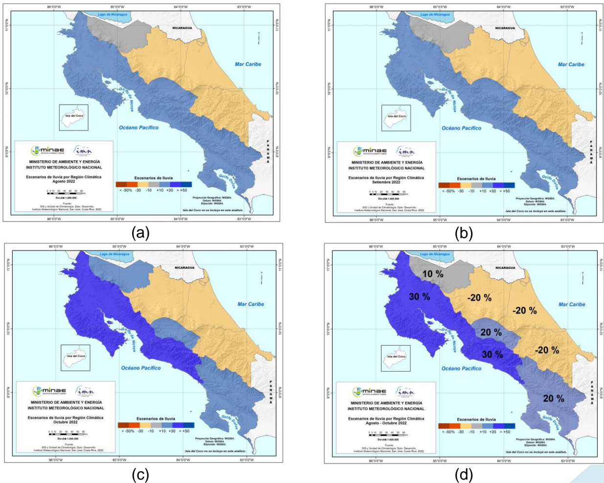
Figura 3. Pronóstico de los porcentajes de lluvia para el periodo agosto a octubre del 2022 (d); así como para los meses de agosto (a), setiembre (b) y octubre (c). Los colores en el mapa indican el escenario de lluvia o sequedad, cuanto más azul es más lluvioso y cuanto más café es más seco en comparación con el promedio. El color gris significa que lloverán los montos normales.
