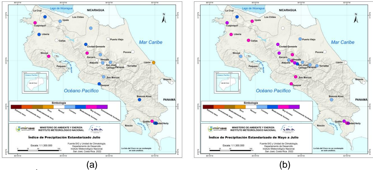
Figura 5. Índice de sequía mensual de julio (a) y trimestral de mayo a julio (b), ambos estimados en base al periodo climático 1991-2020. Las tonalidades de los colores de colores azul y morado se asocian a condiciones de excedente de lluvia; mientras las tonalidades de los colores café y rojo se asocian a condiciones deficitarias de lluvia.
