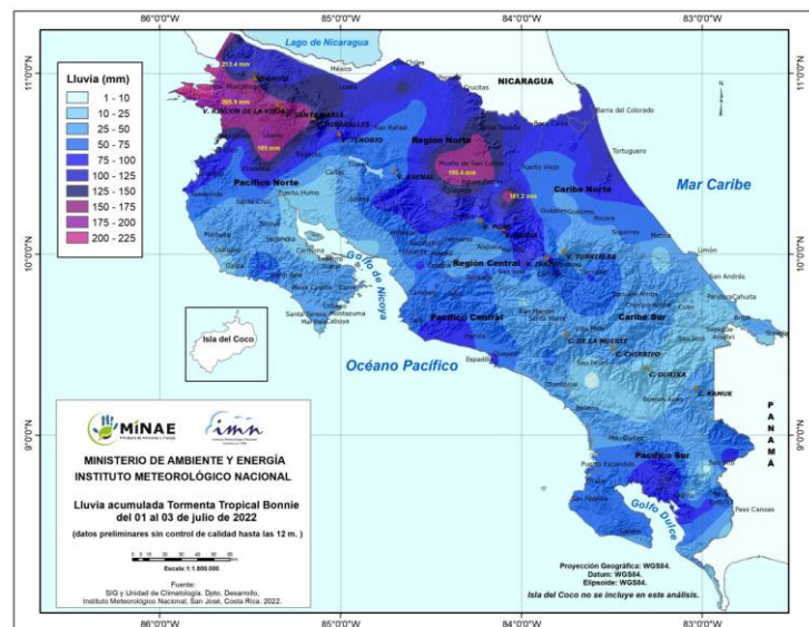
Figura 1.1. Mapa de lluvia acumulada debido a la tormenta tropical Bonnie del 1 al 3 de julio del 2022.
